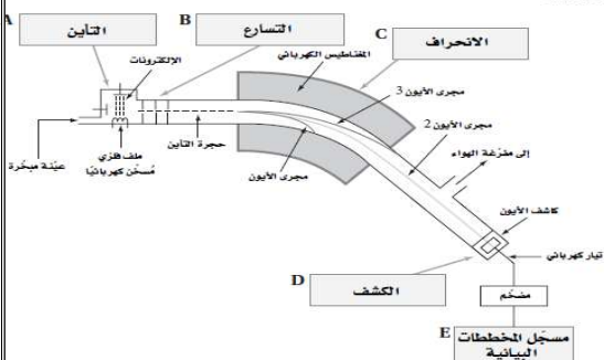
مطياف الكتلة
